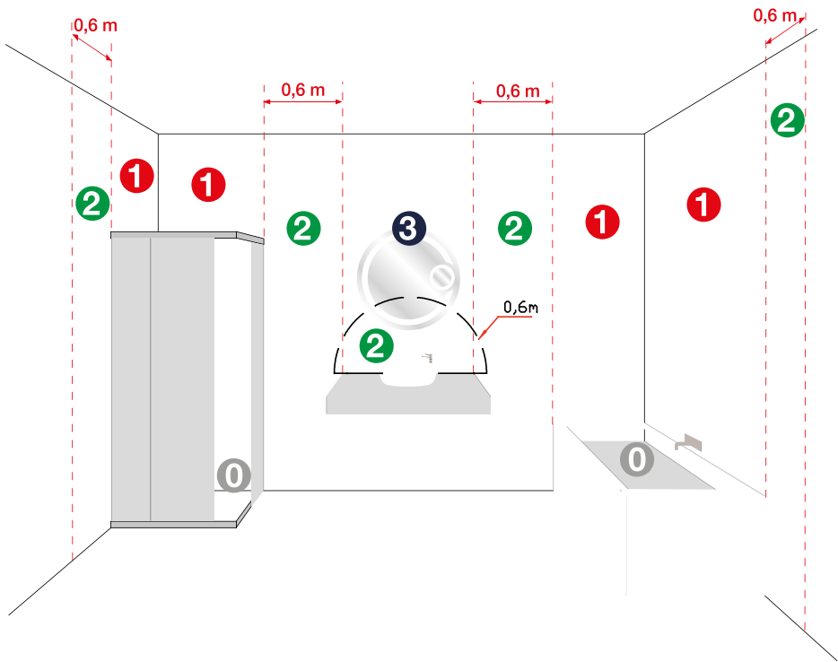
DISTANZE DI SICUREZZA - INSTALLATION SAFETY DISTANCES
